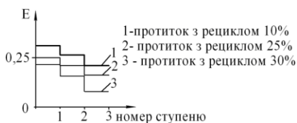
Рисунок 7 – Вплив способу рециркуляції сушильного агента на ефективність процесу сушіння
