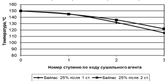
Рисунок 11 – Вплив способу байпасування сушильного агента на зміну температури сушильного агента
