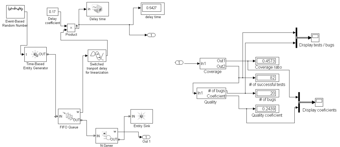
Рисунок 2 – Випробовування моделі процесу тестування для модуля В: коефіцієнт покриття та коефіцієнт якості
