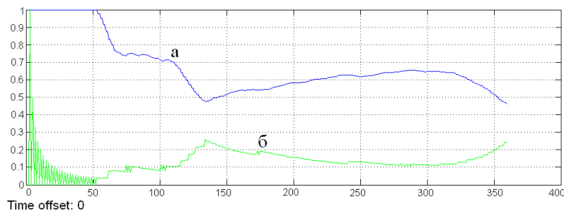
Рисунок 4 – Випробовування моделі процесу тестування для модуля В: коефіцієнт покриття (а) та коефіцієнт якості (б)
